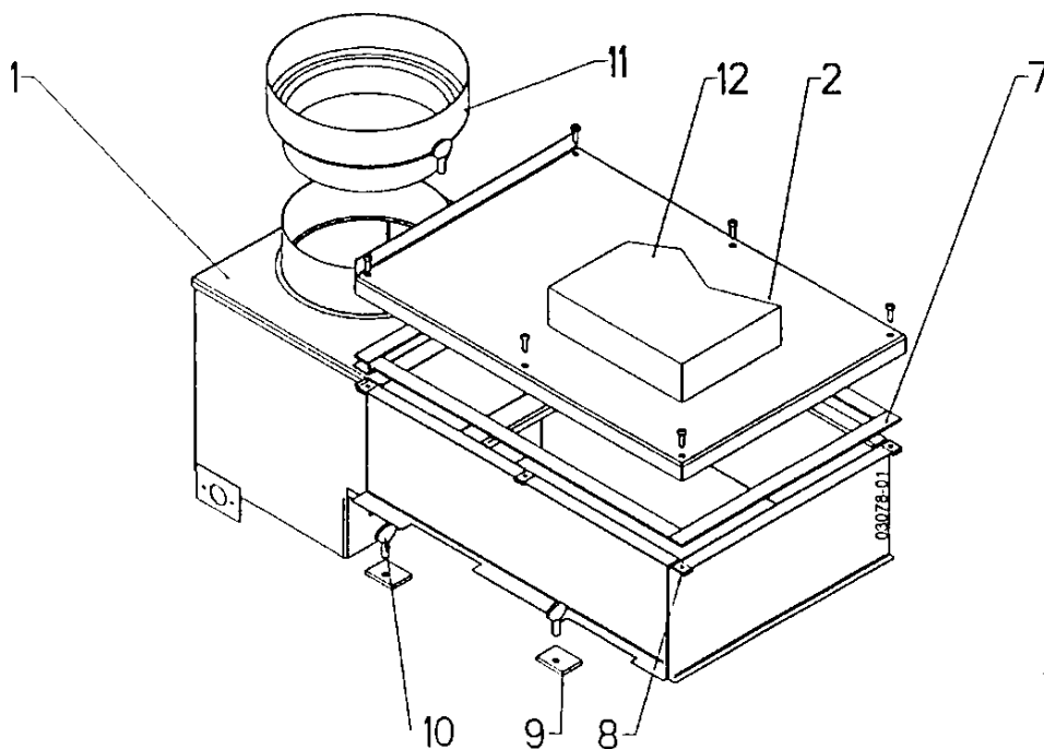
Ensemble boîte à fumées 5 à 7 éléments
