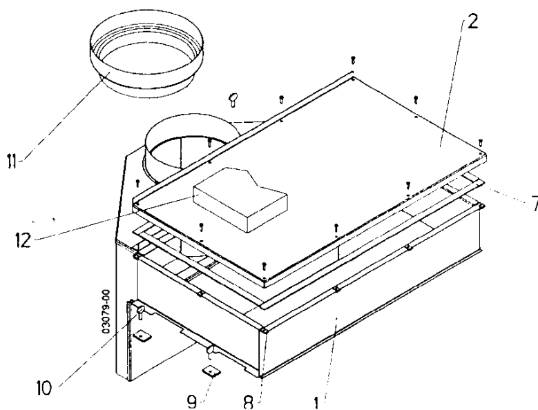
Ensemble boîte à fumées 8 à 22 éléments
